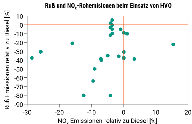
Abbildung 2: Übersicht über Emissionen beim Einsatz von HVO im Vergleich zu Diesel. Verwendet wurden Ergebnisse von Motoren unterschiedlicher Bauart (LKW und PKW) in diversen Betriebspunkten. Eigene Darstellungen mit Daten aus [1–6]
